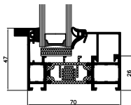
Querschnitt durch feststehendes Fenster
